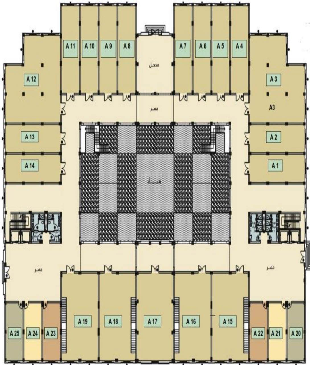
المسقط الأفقي للدور الأرضي
